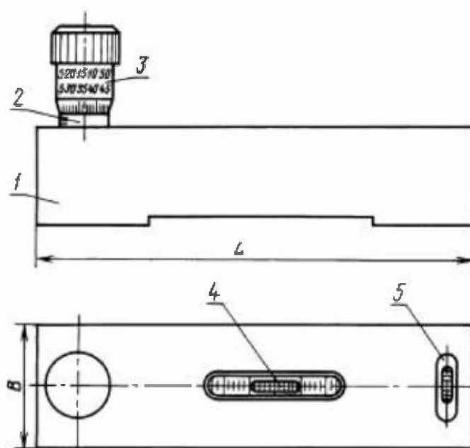
1 — основание; 2 — стебель; 3 — барабан; 4 — продольная ампула; 5 — поперечная ампула
