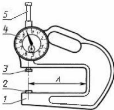
1 — корпус; 2 — планка; 3 — измерительный наконечник; 4 — отсчетное устройство; 5 — измерительный стержень; A — вылет
