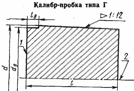
1—измерительная плоскость; 2—ось калибра Черт. 3
