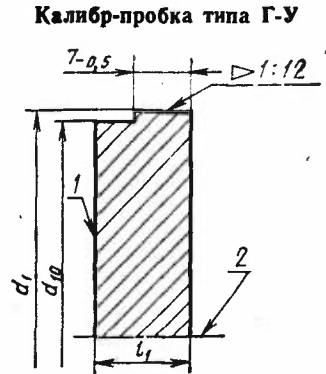
1—измерительная плоскость; 2—ось калибра Черт. 4
