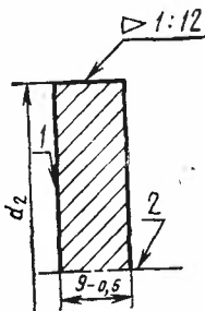
1—измерительная плоскость; 2—ось калибра Черт. 5
