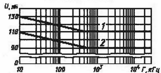
Предельные значения напряжения гармонических помех в полосе частот от 10 кГц до 30 МГц
