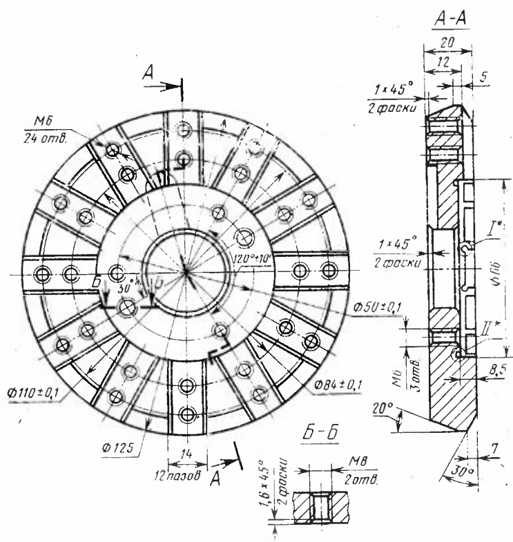
Корпус (поз. 1)
